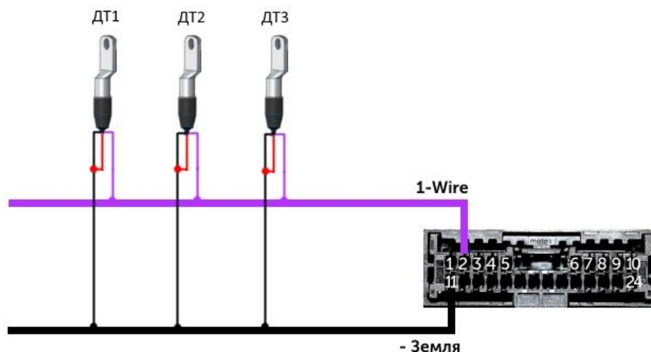
Рис. 4.1. Схема подключения датчиков температуры к шине 1-Wire.
