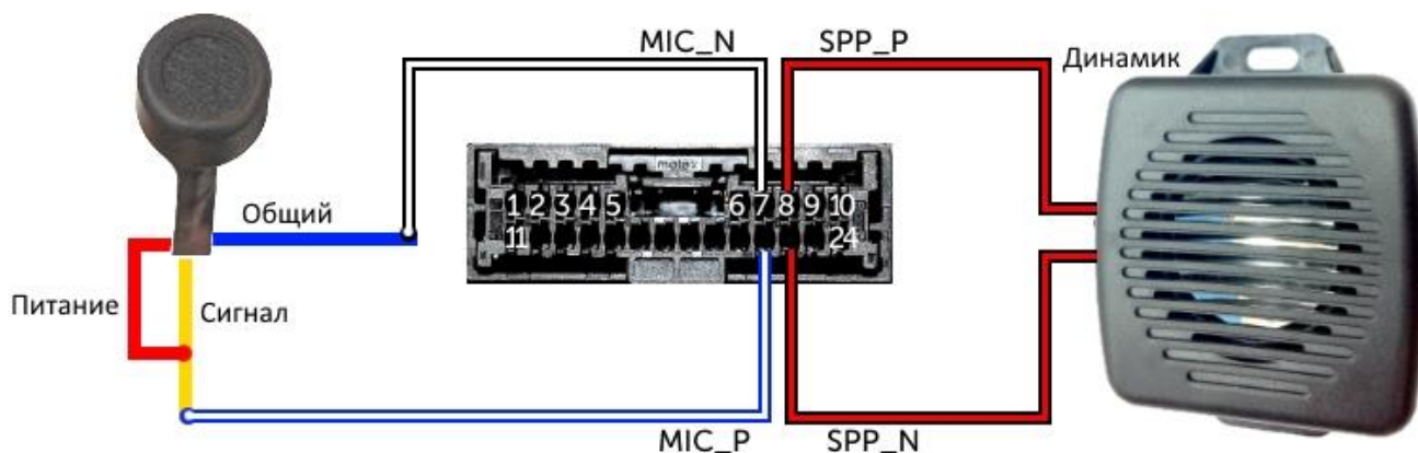
Рис. 4.7. Схема подключения микрофона и динамика.
